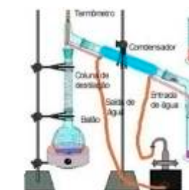
Aparelho Destilador de Asfalto Diluido, com ou sem termômetro (sob medida).
